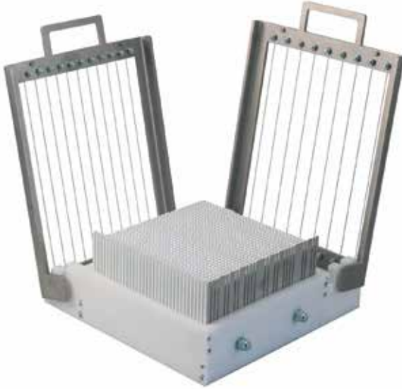
Gitar Çiftli Dilimleme Makinası Double Guitar
